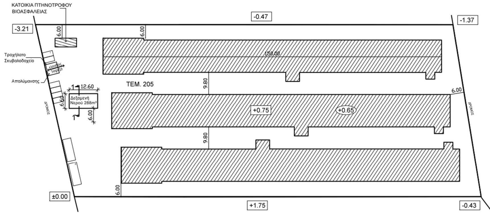
Εικόνα 3: Χωροταξικό Προτεινόμενης Μονάδας
