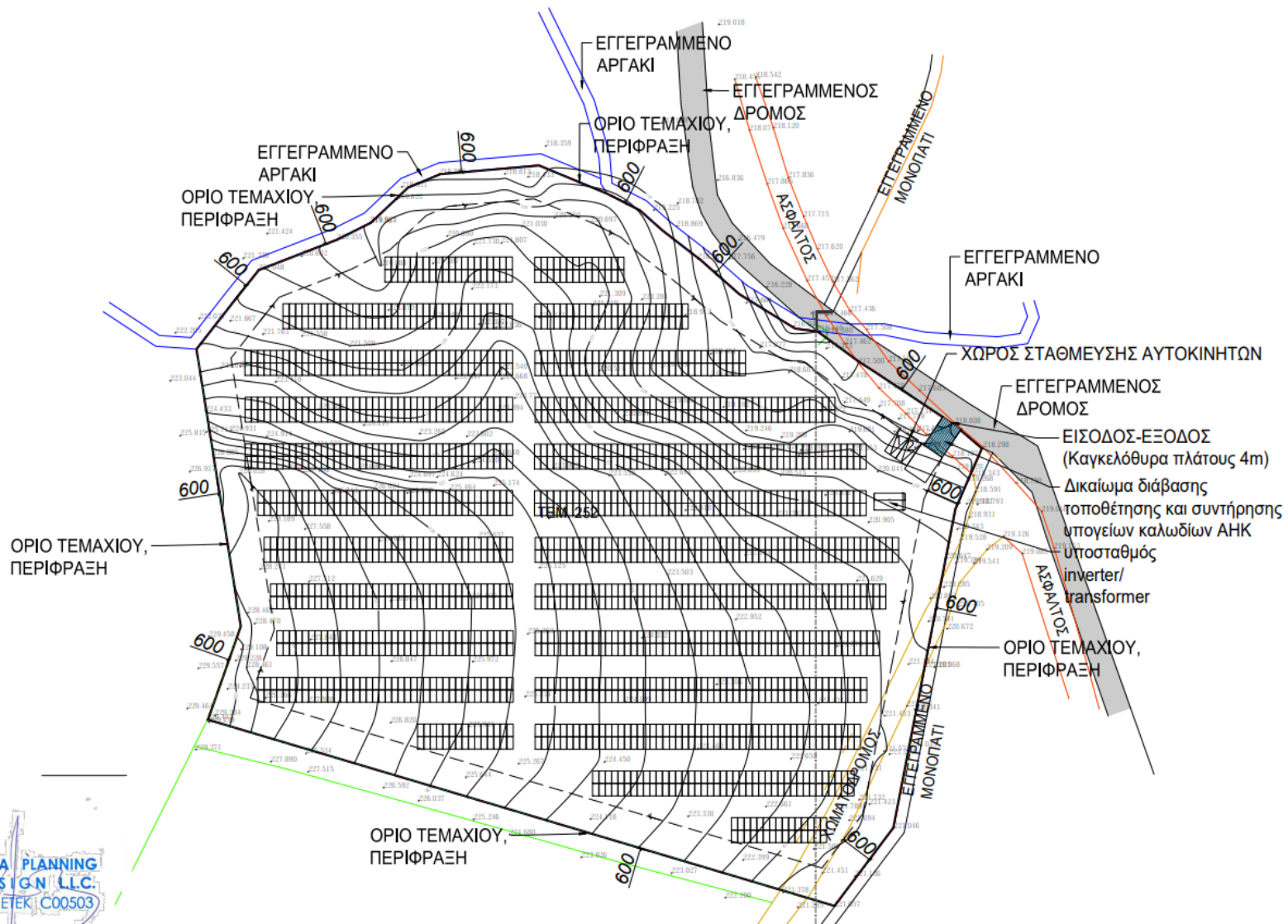
Εικόνα 4: Χωροταξικό Σχέδιο προτεινόμενου φωτοβολταϊκού πάρκου
