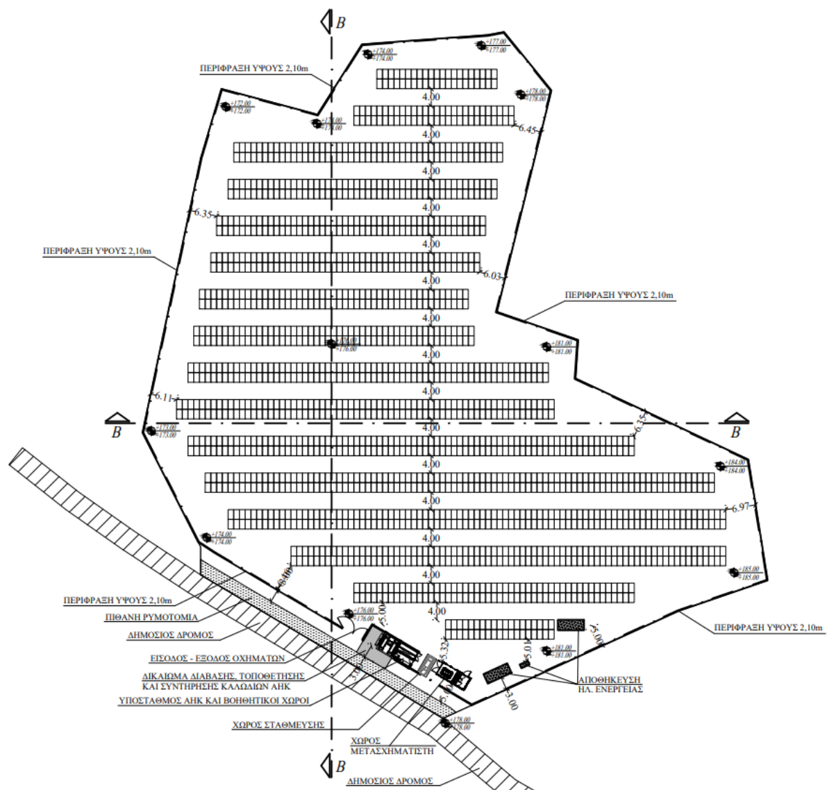
Εικόνα 4: Χωροταξικό Σχέδιο προτεινόμενου φωτοβολταϊκού πάρκου
