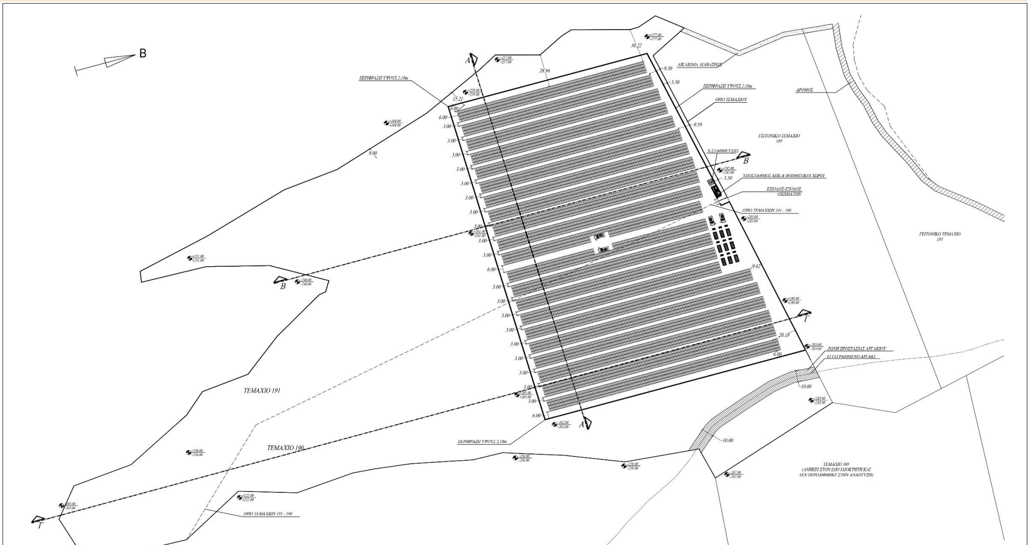
Εικόνα 4: Χωροταξικό Σχέδιο προτεινόμενου φωτοβολταϊκού πάρκου
