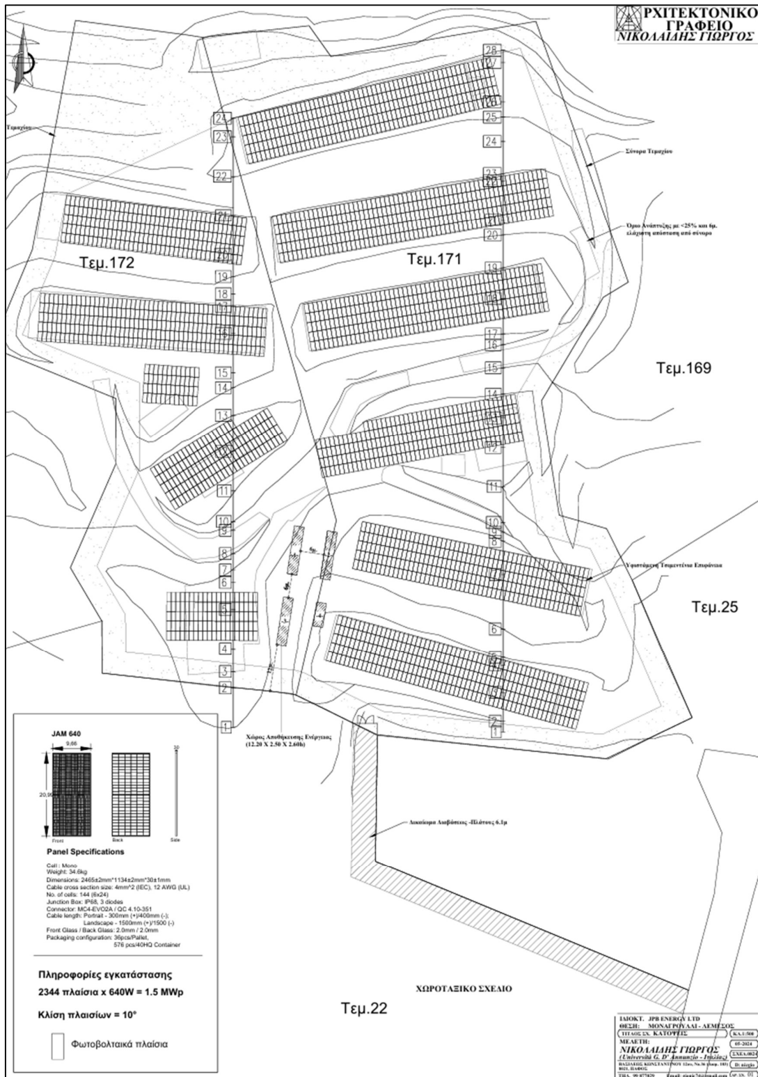
Εικόνα 4: Χωροταξικό Σχέδιο προτεινόμενου φωτοβολταϊκού πάρκου
